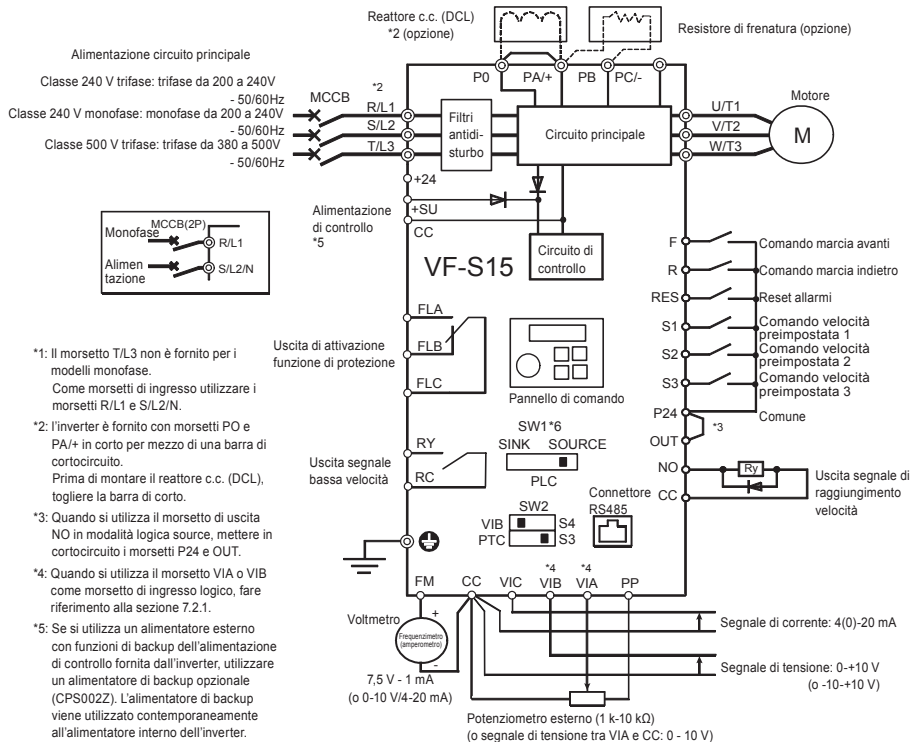
Schema di connessione standard - SOURCE (positiva) (comune: P24)
